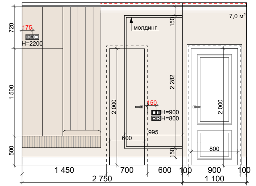
Разрез 4-4
