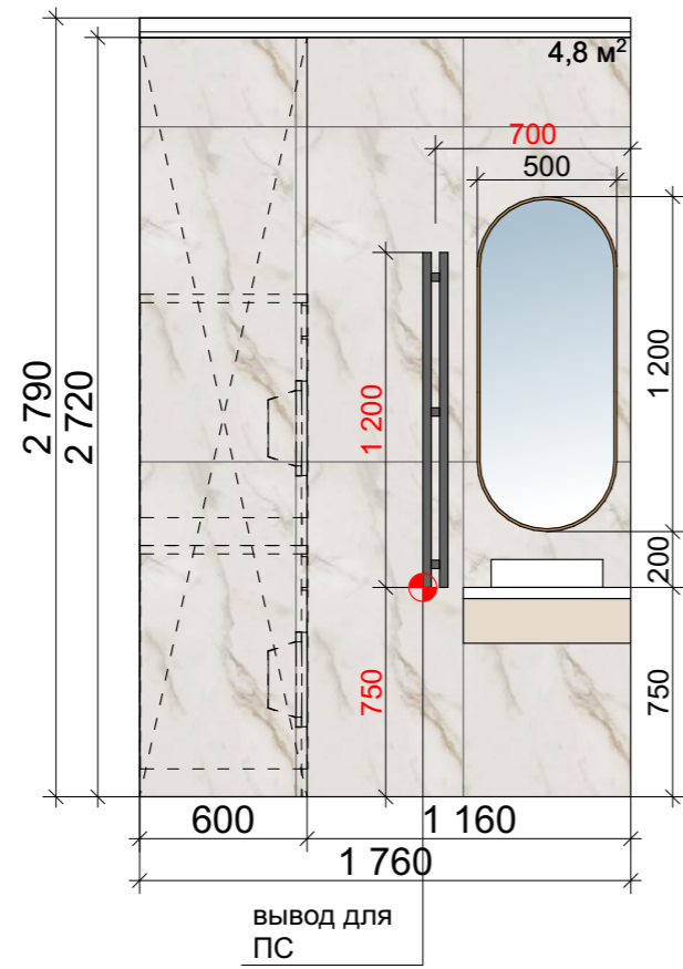
Разрез 1-1
