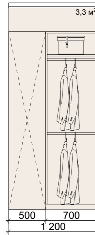
Разрез 3-3
