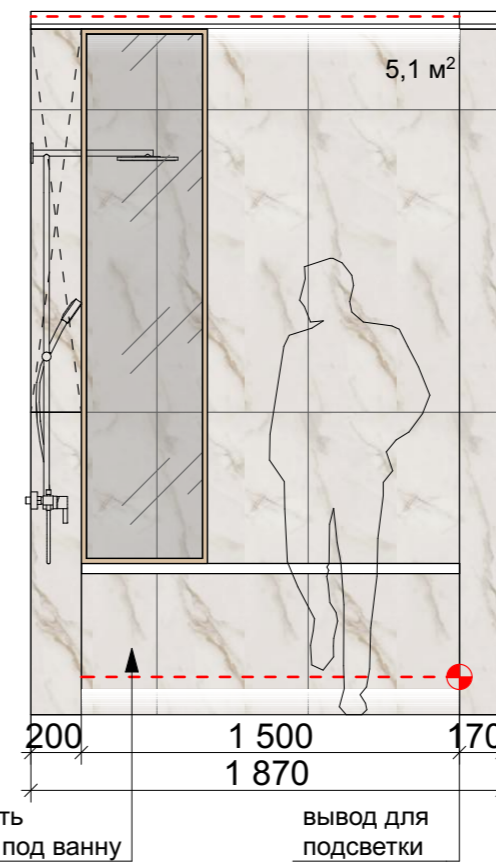
Разрез 3-3
