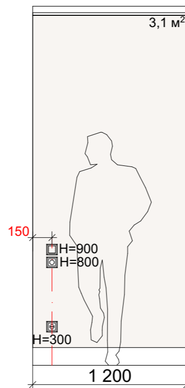
Разрез 2-2
