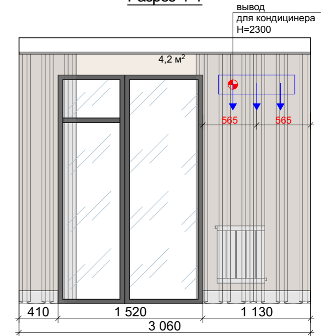
Разрез 4-4
