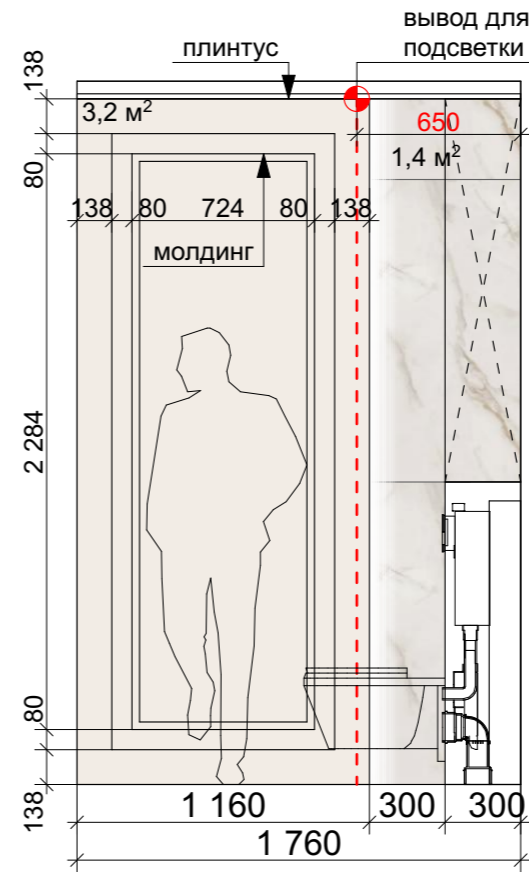
Разрез 3-3
