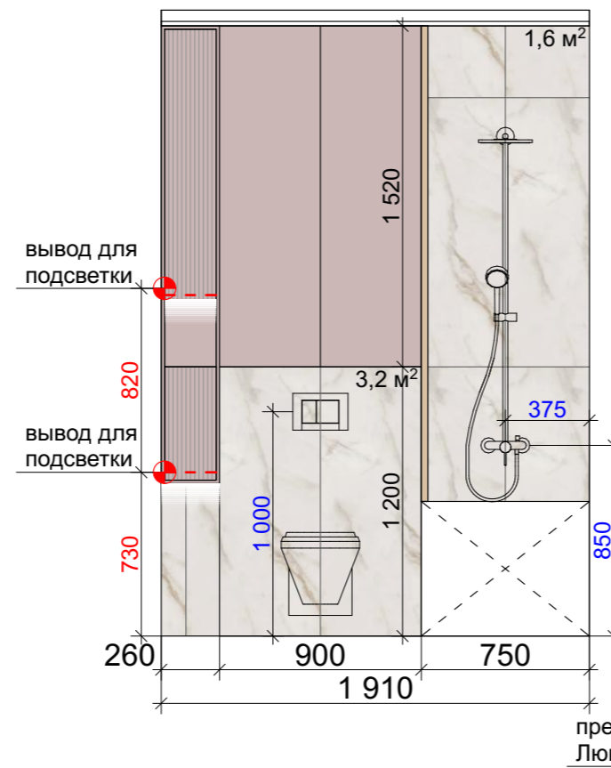
Разрез 2-2
