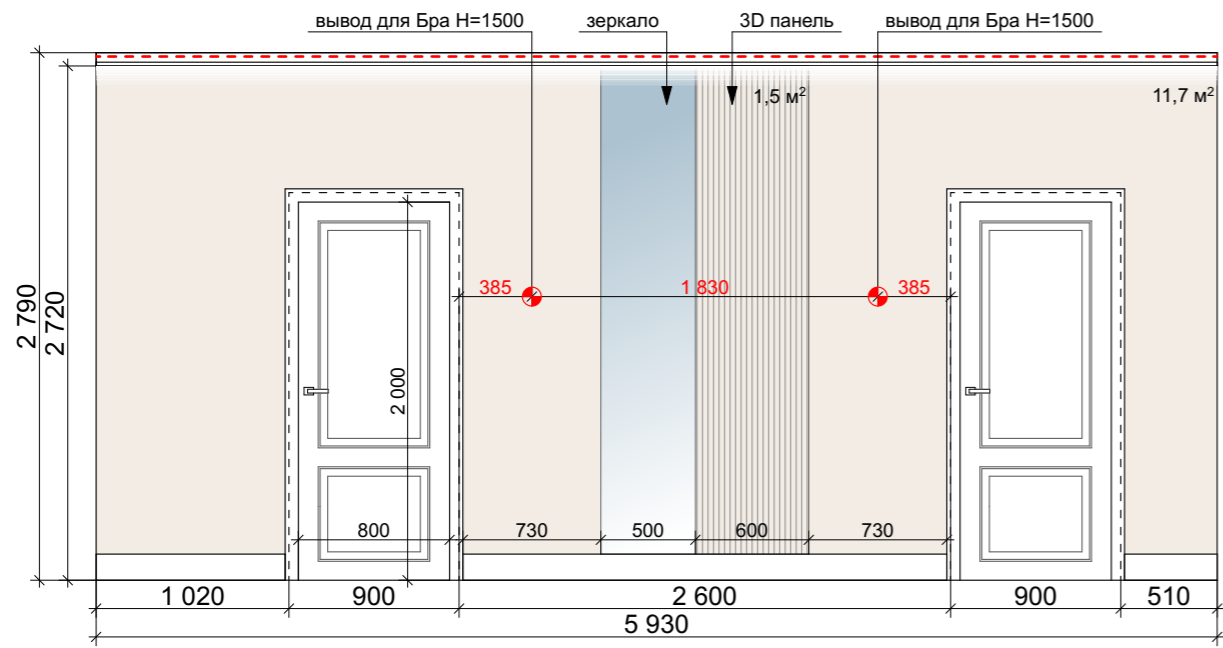
Разрез 1-1
