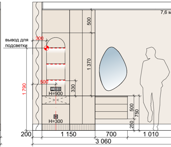
Разрез 2-2
