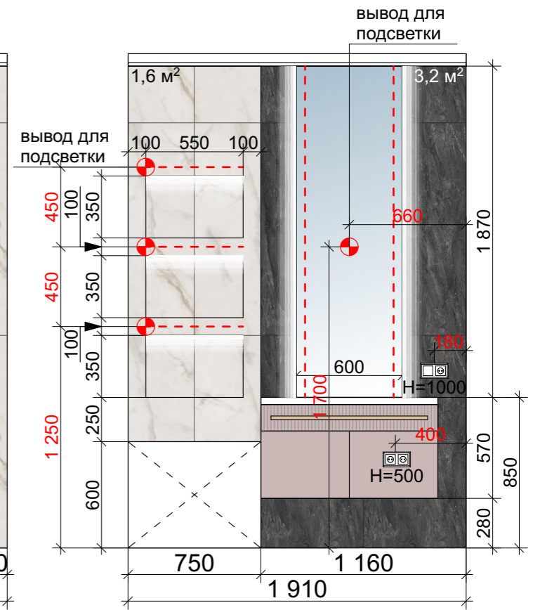
Разрез 4-4
