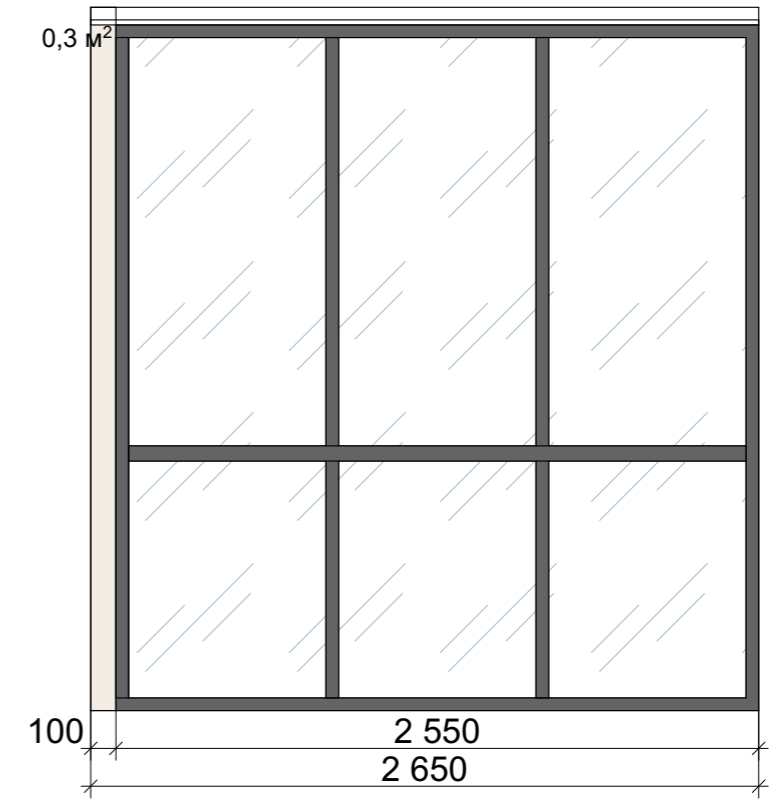
Разрез 4-4
