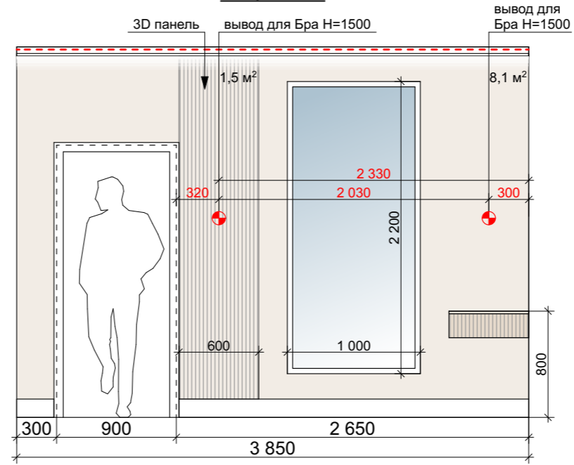
Разрез 2-2
