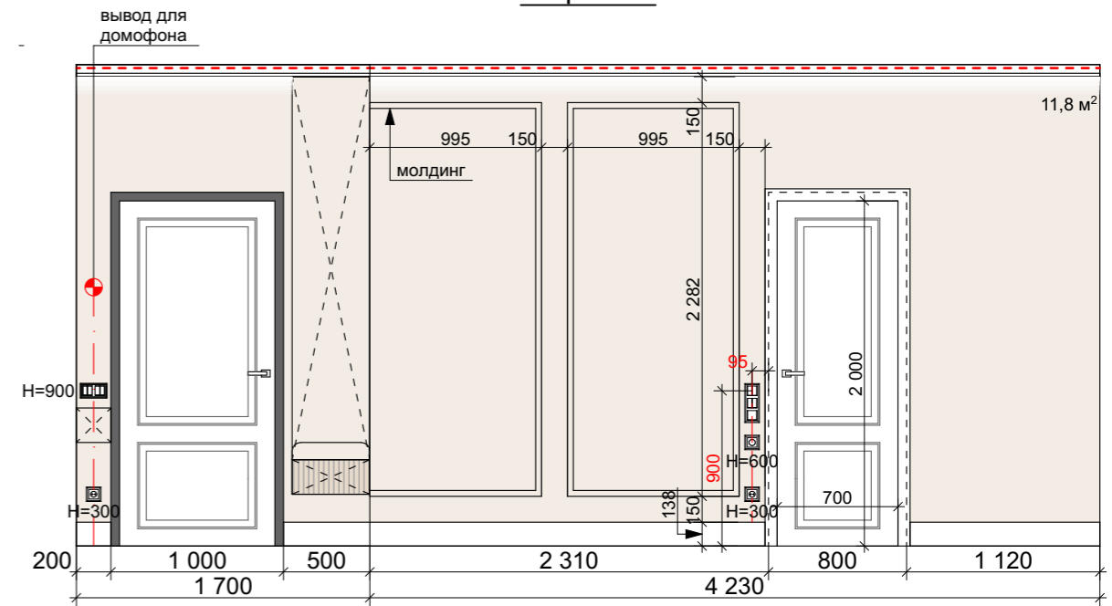
Разрез 3-3
