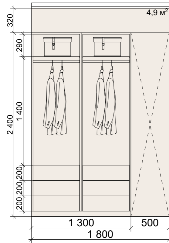
Разрез 2-2
