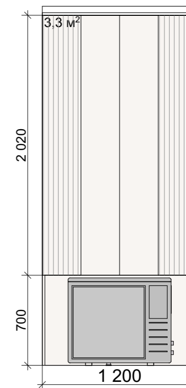
Разрез 4-4
