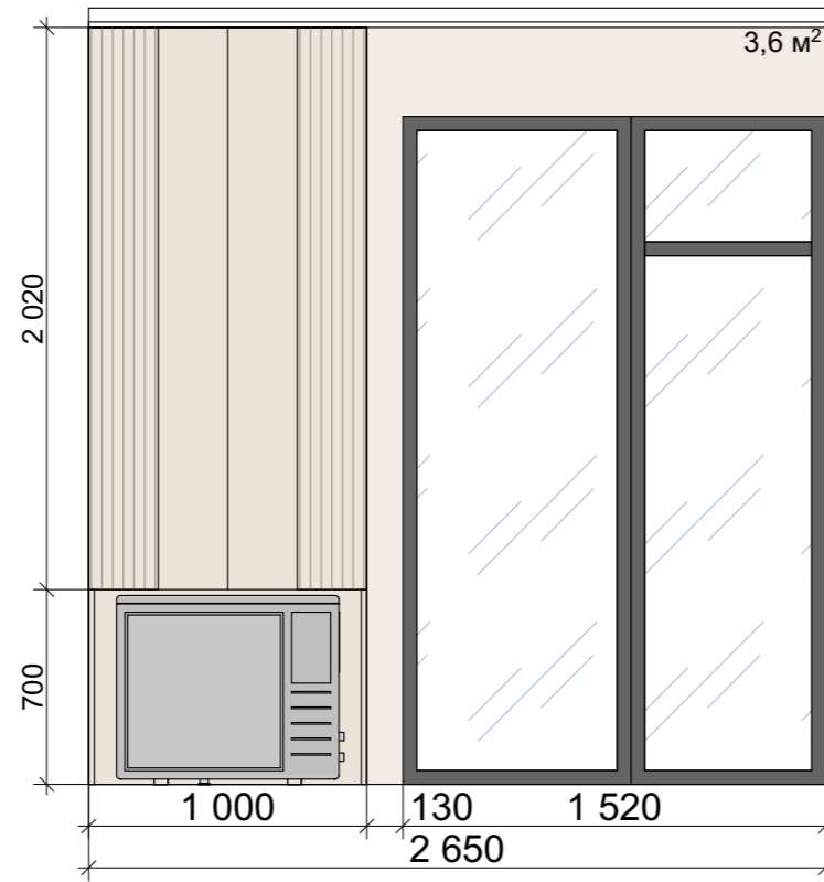
Разрез 2-2
