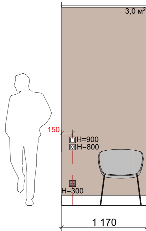
Разрез 3-3
