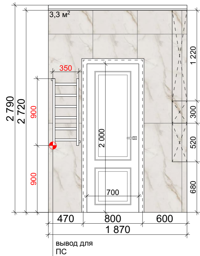
Разрез 1-1
