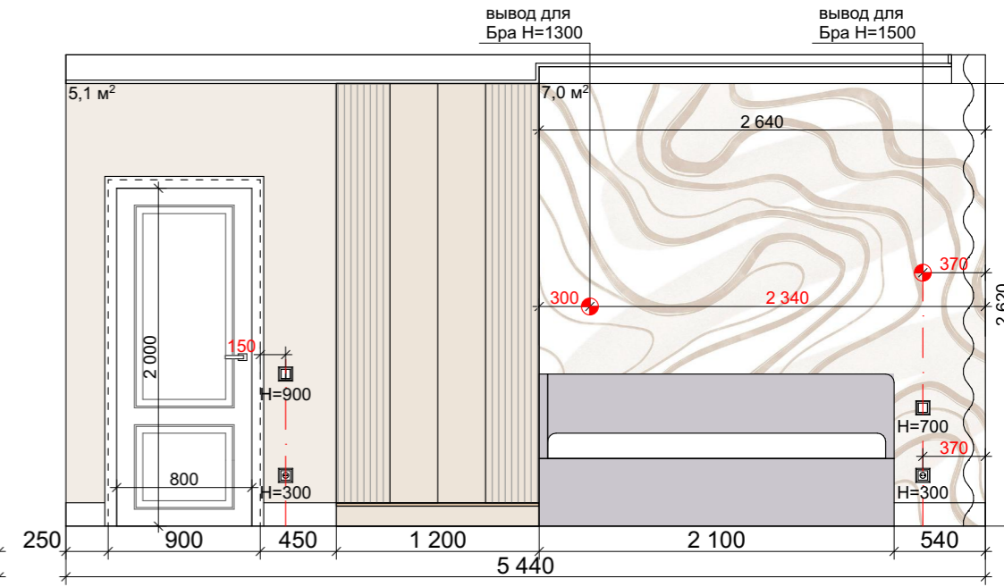
Разрез 3-3
