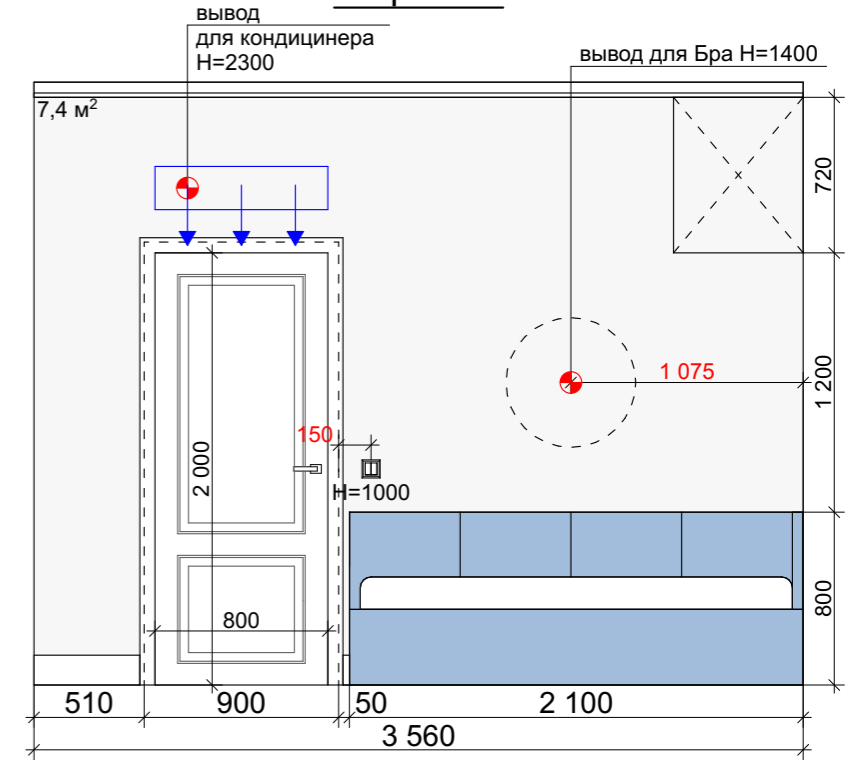
Разрез 3-3
