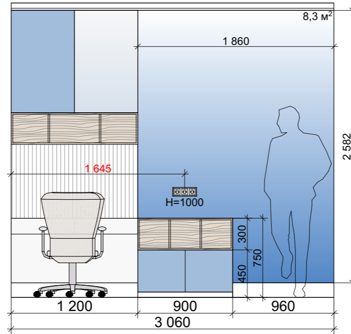
Разрез 2-2
